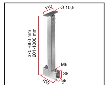
KATTOKANNATIN KKS-100 370-600mm/601-1000 mm, säädettävä
