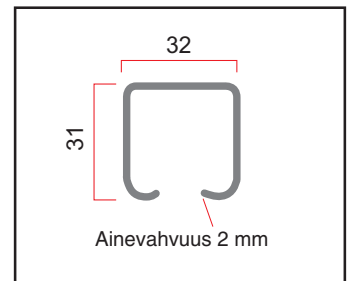
KISKO K-100 Kantavuus 100 kg, vakio pituus 6 m
