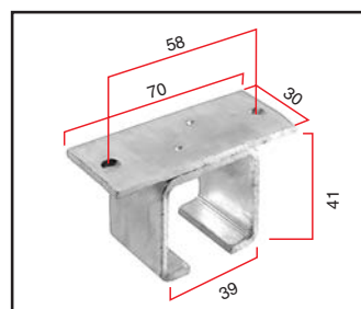
KATTOKANNATIN KKK-100 Kiinteä
