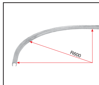
KAARI 90°, säde 600 mm
